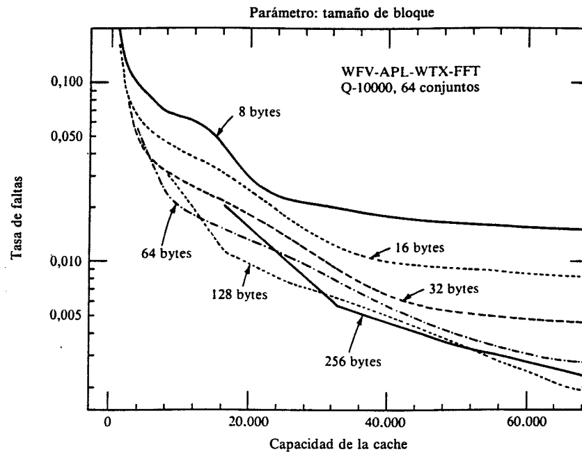
(a) Tamaño de cuanto, Q = 10.000 referencias
