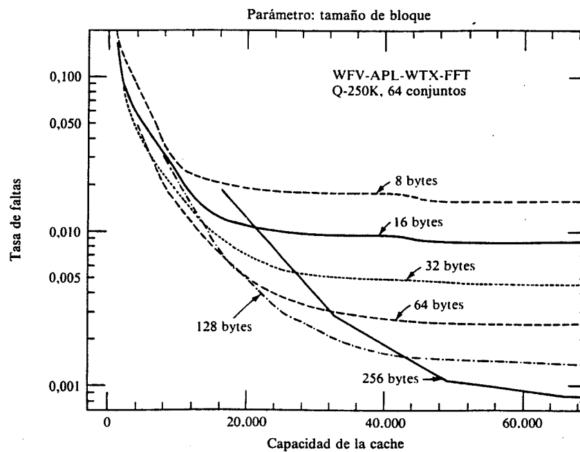
(b) Tamaño de cuanto, Q = 250K referencias
