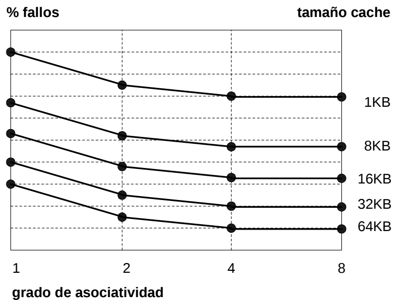
Gráfica 2. Ejemplo de comportamiento de una memoria cache con 32 bytes de tamaño de bloque ante cambios del grado de asociatividad
