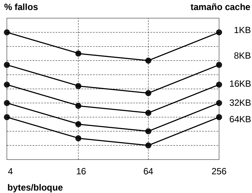
Gráfica 1. Ejemplo de comportamiento de una memoria cache de correspondencia directa ante cambios del tamaño de bloque
