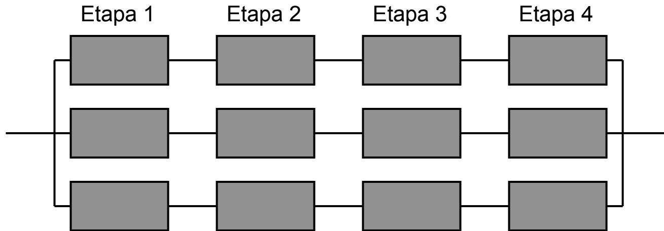
Cauce superescalar de orden 3
